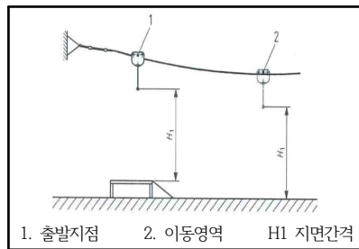
[그림 3] 매달림형 공중 놀이기구의 지면간격 측정
